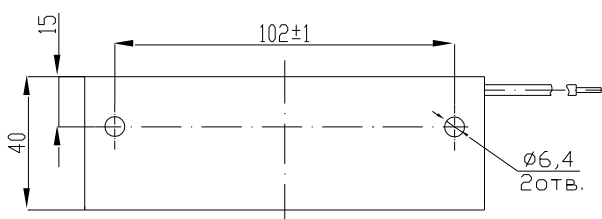
Блок геркона
