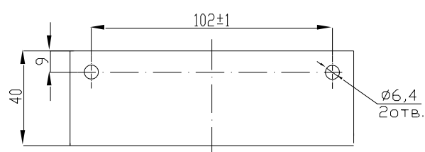
Блок магнита
