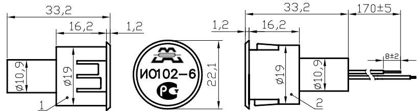
Рис 1. Габаритные и установочные размеры извещателя
