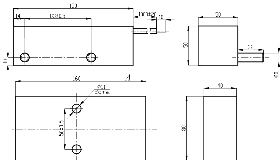
Рисунок 3. Габаритные и присоединительные размеры извещателя
